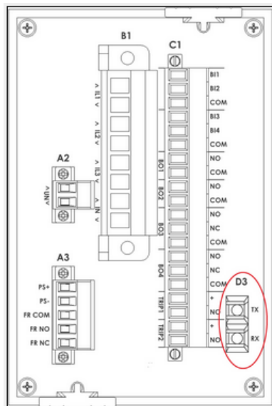
Figure 1.1.2 : Panneau arrière de l'appareil S16, indiquant le port de communication série
